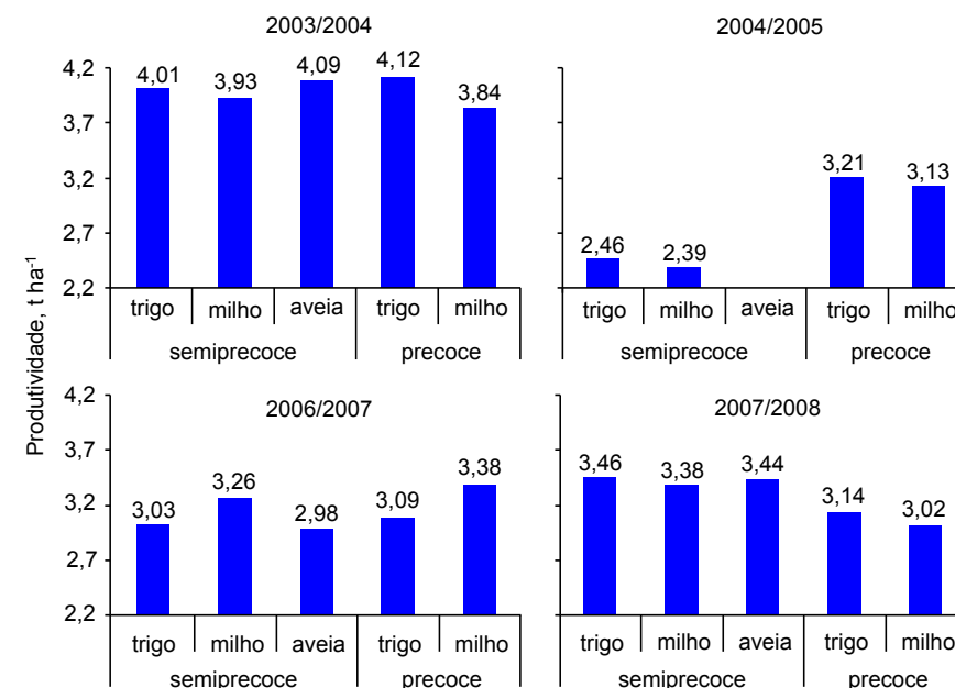
Figura 6. Produtividade de cultivares de soja de diferentes ciclos em sistemas de rotação de culturas. Semiprecoce: ciclo aproximado de 125 dias; precoce: ciclo aproximado de 118 dias. De acordo com o sistema de rotação de culturas, a soja pode ser cultivada após trigo, milho ou aveia no inverno. Embrapa Soja/Coamo, Campo Mourão/PR, 2008.
