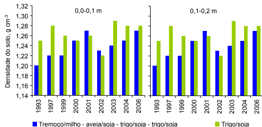
Figura 1. Densidade de um Latossolo Vermelho distroférico manejado sob SPD, em função do sistema de culturas, da época e da profundidade de amostragem. Embrapa Soja, Londrina/PR, 2010.
